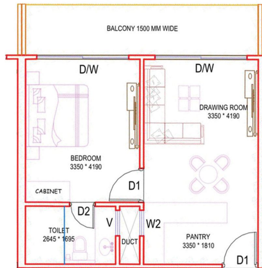
1BHK -LAYOUT
